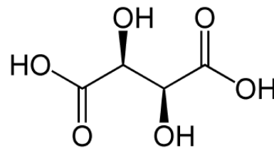
Strukturformel Weinsäure
