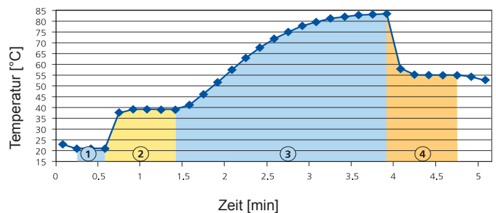
Temperaturprofil eines Dekontaminationsprozesses für Behälter mit menschlichen Ausscheidungen
